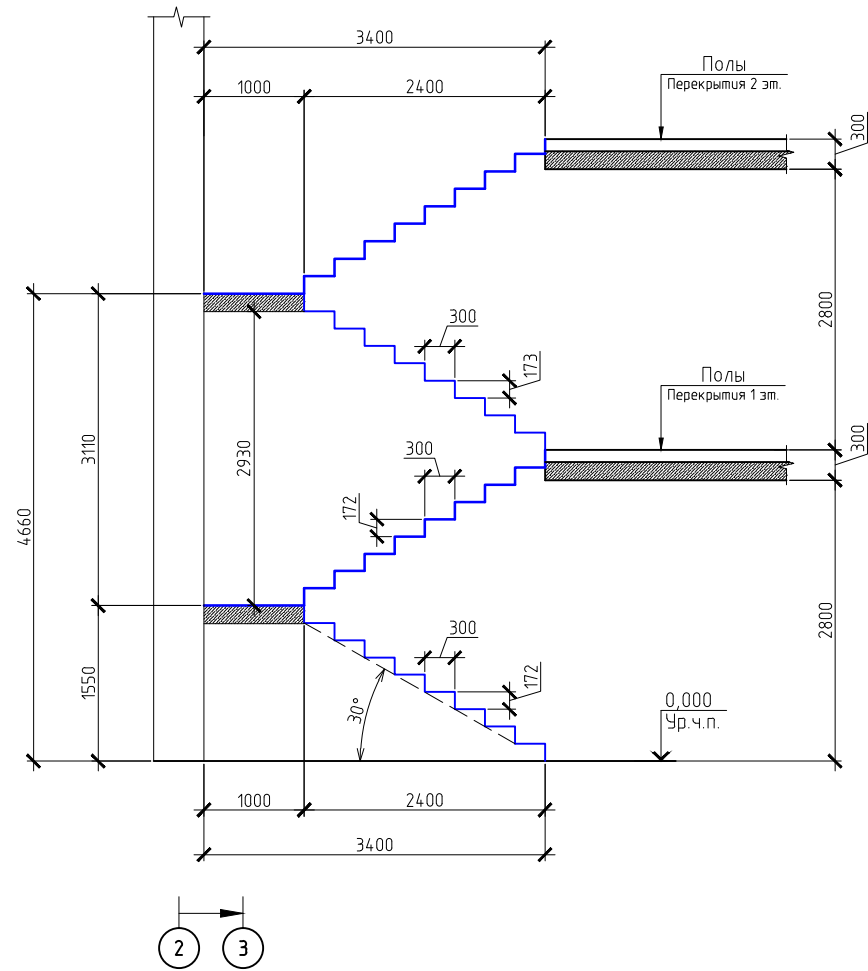
Схема ступеней монолитных ж/бетонных лестничных маршей. Продолжение.
